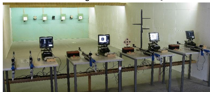
Bestehende 10m Luftgewehranlage mit 4 elektronischen Scheiben
